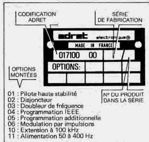
Figure 3-1 : CARACTERISATION DU GENERATEUR
