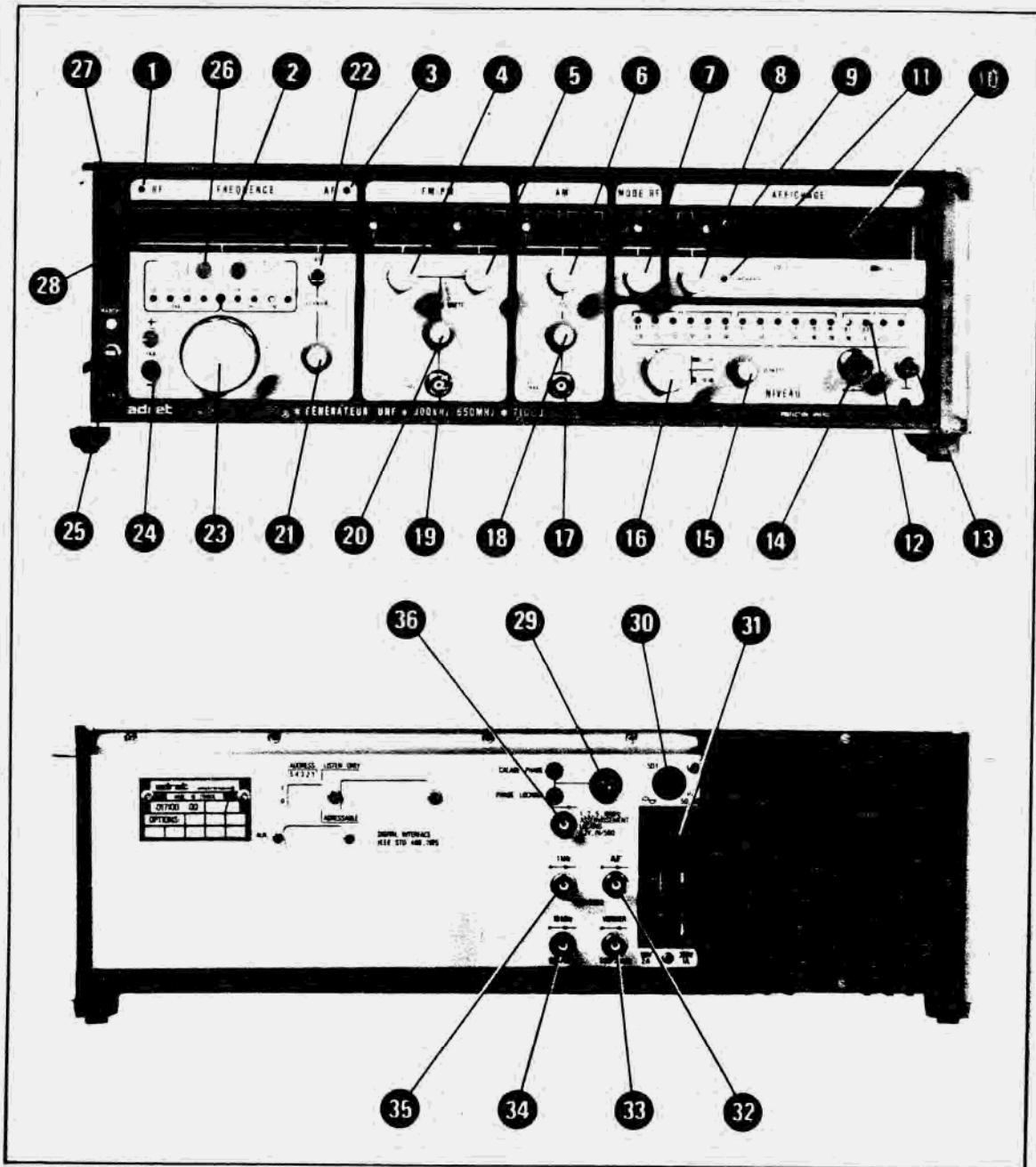
FIGURE 3 - 4 : LOCALISATION des commandes de la VERSION DE BASE
